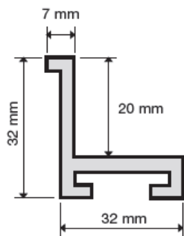
Dettaglio profilo telaio
